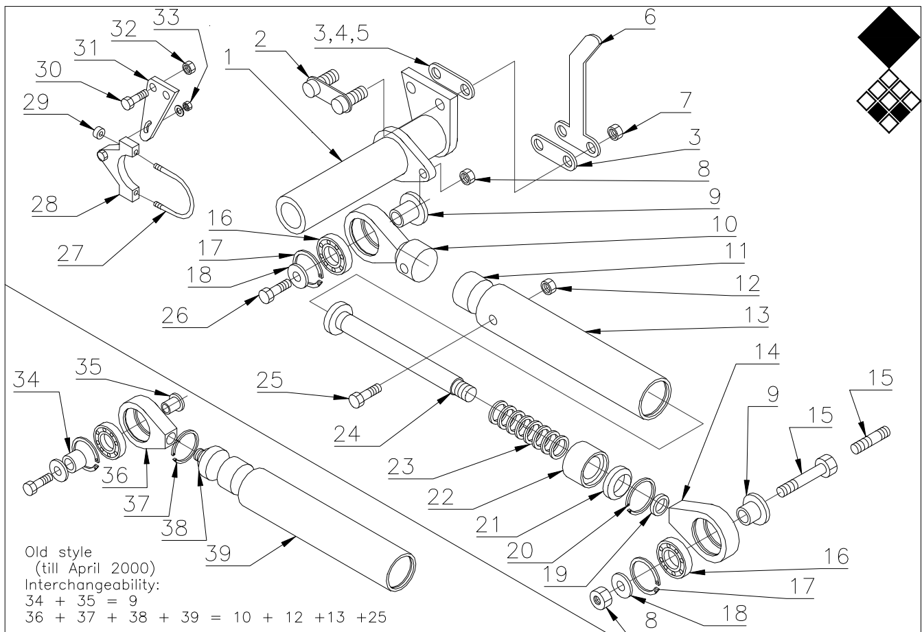
Redexim-Charterhouse Verti-Drain 7316 pag 04-1 code 1004
