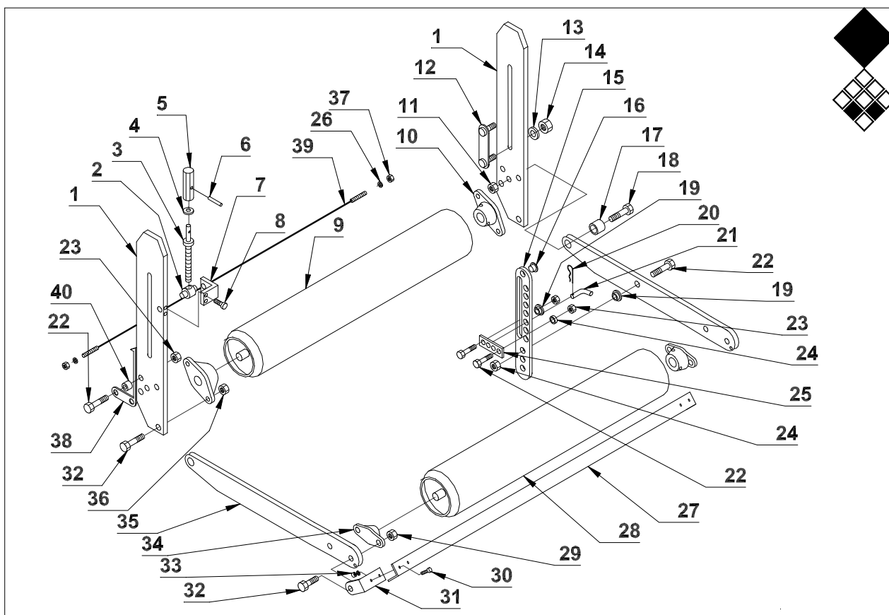
Redexim-Charterhouse Verti-Drain 7316 pag 09 code 0718
